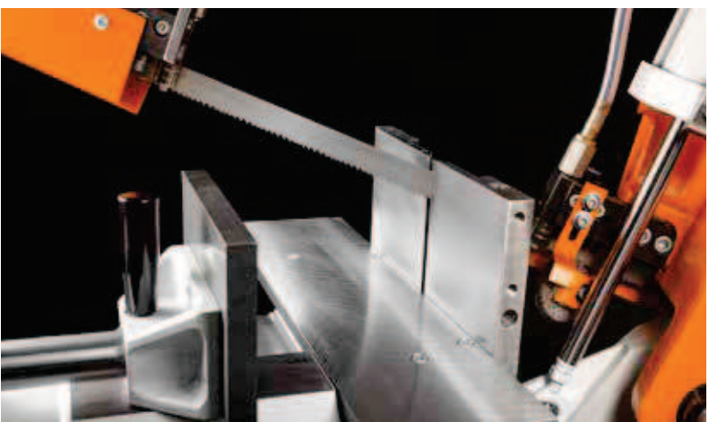
Beidseitig geschlossene Rillenkugellager und Hartmetall-Sägebandrücken-Gleitführung.
